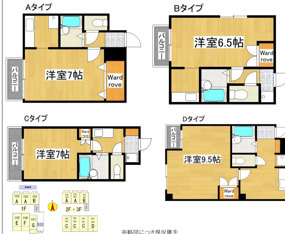
【間取り図】
